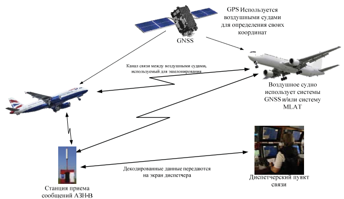
Рис. 2. Общая схема приема-обработки сигналов АЗН-В
