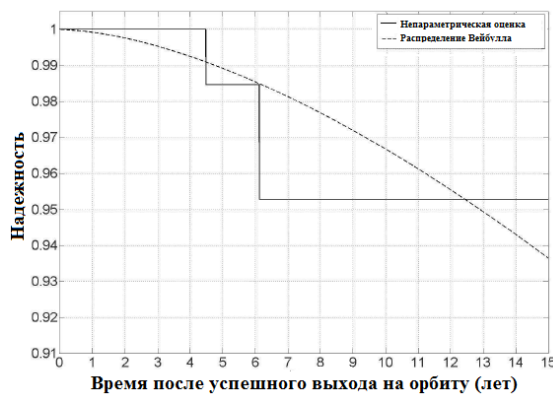
Средняя околоземная орбита
