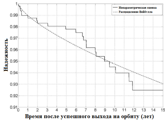
Геосинхронная орбита
